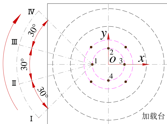
图 10 第三级荷载加载方式
