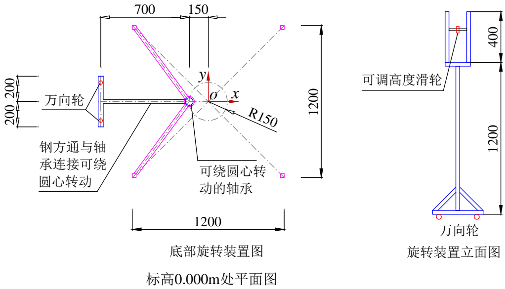
附图3 加载台平立面图
