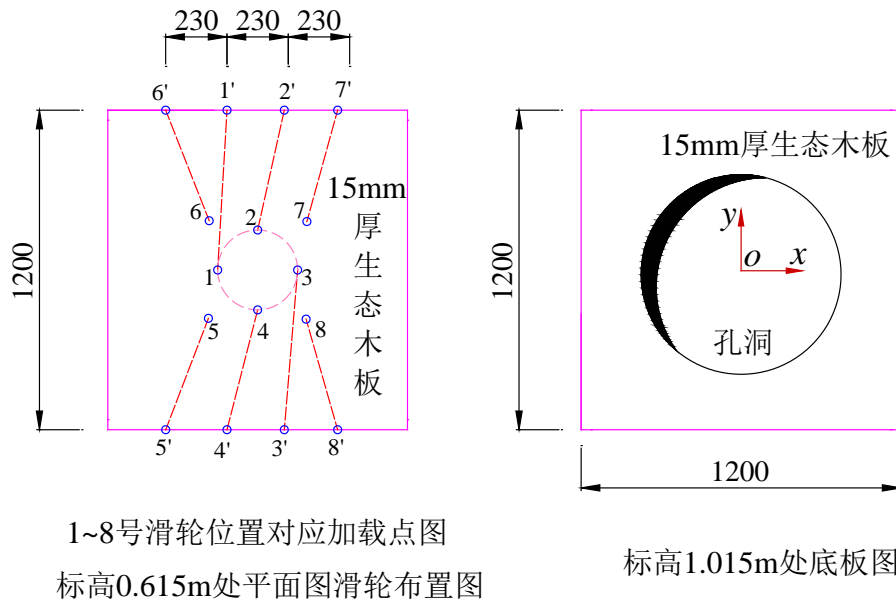
附图4 滑轮位置布置图及模型底板图
